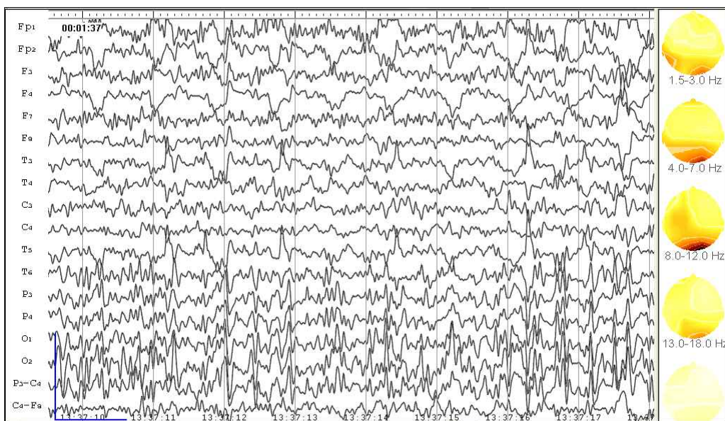
Диаграмма2. Волонтер находится под действием торсионного поля базовой станции, на которой установлена защита.
