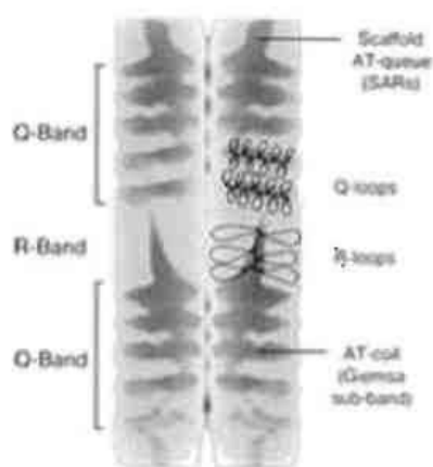
Рис. 5. Метафазная модель хромосомы [8].
