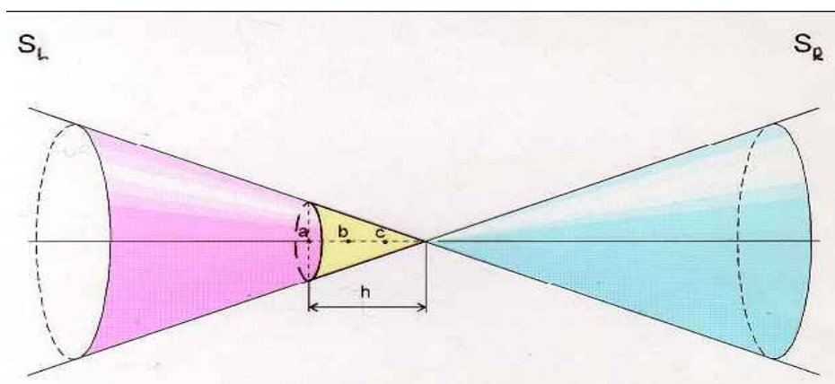
Рис. 9-а ТП цилиндра.
