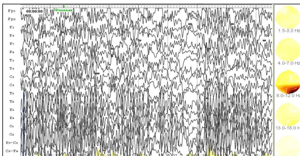
Диаграмма 1. Волонтер находится под действием торсионного поля базовой станции
