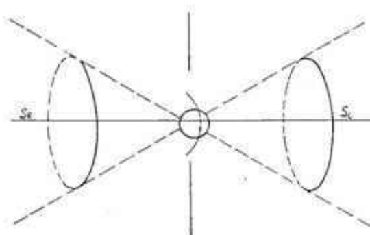
рис. 5. Диаграмма направленности торсионного поля объекта со спином
